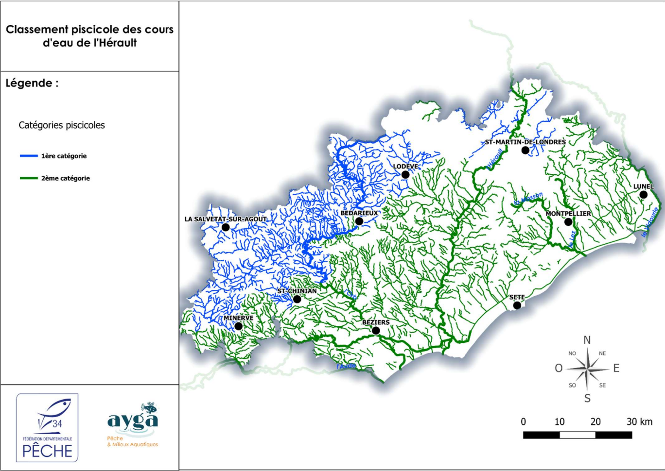
Figure 41 : Catégories piscicoles des cours d'eau de l'Hérault
