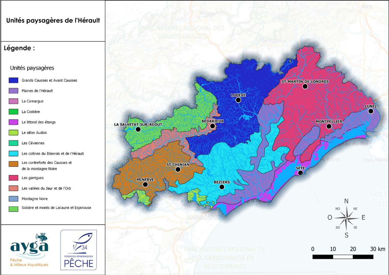
Figure 2 : Entités paysagères de l'Hérault
