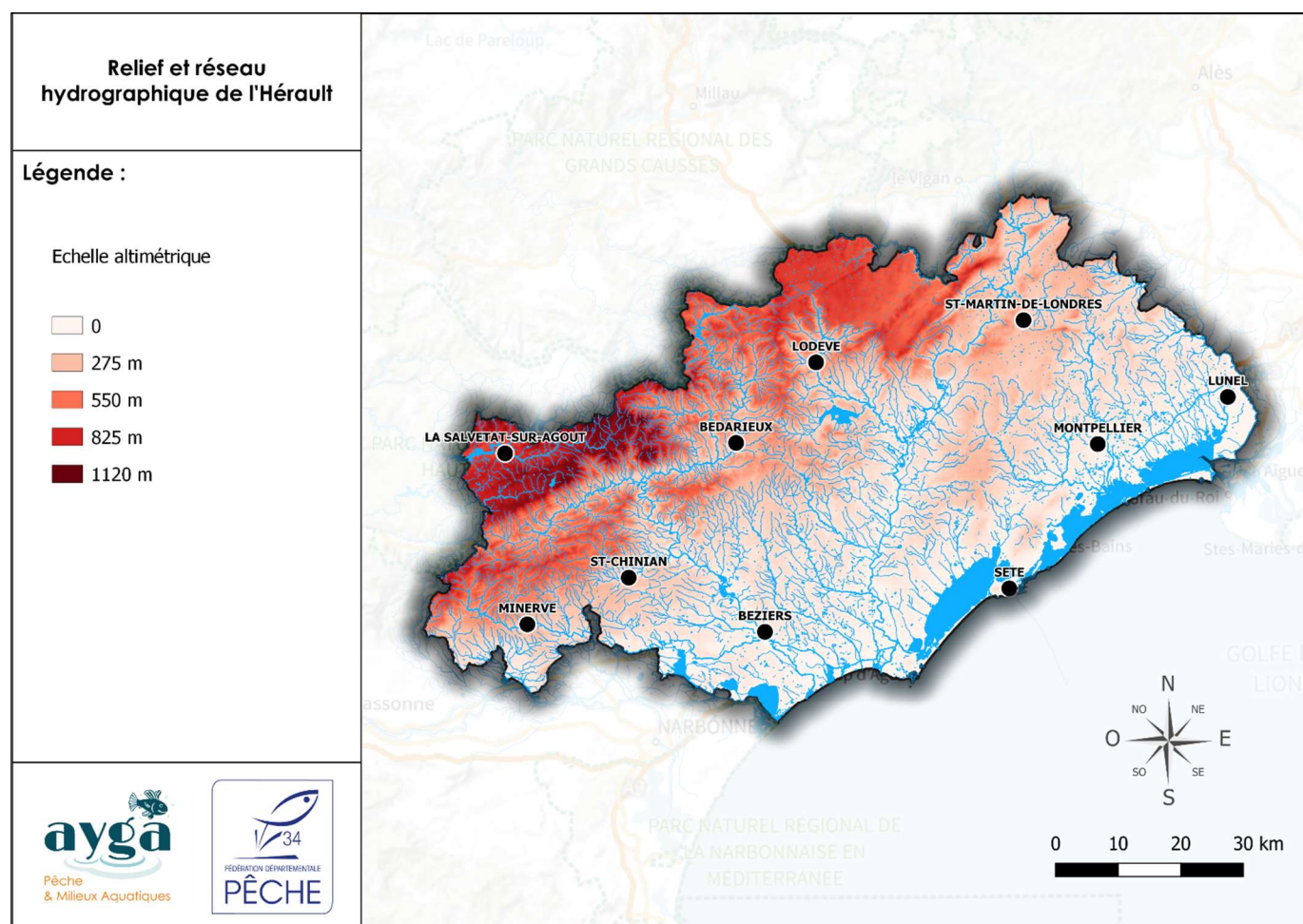
Figure 3 : Relief réseau hydrographique de l'Hérault
